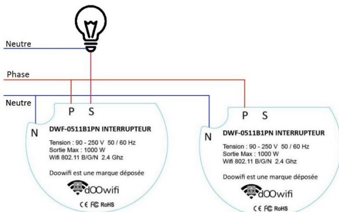
VA-ET-VIENT PAR SCENARIOS ENTRE 2 INTERRUPTEURS
